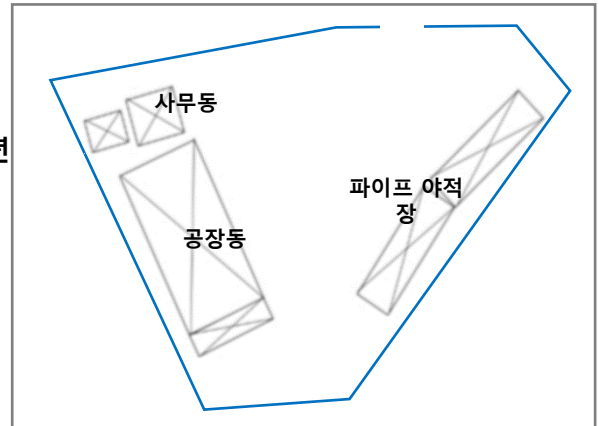
▲ 공장 배치도
